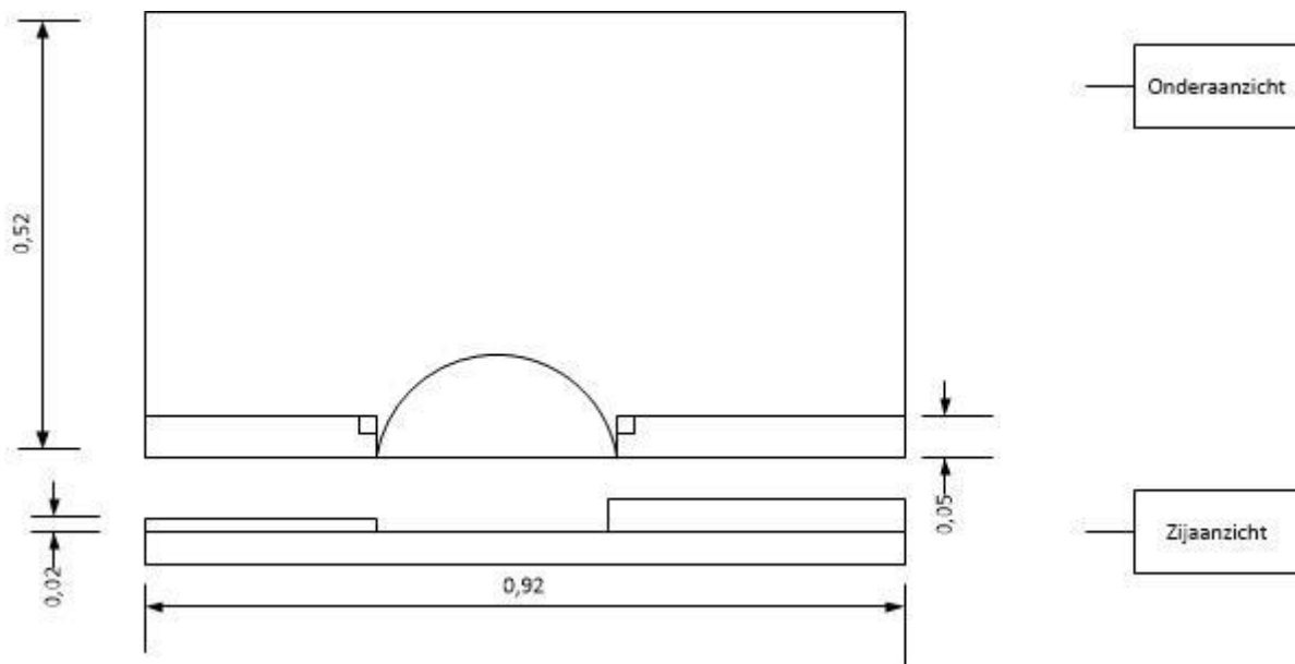
afb. 10 Tekening hulpstuk
